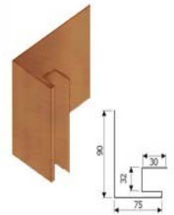
Откос 75 x 90 см.
