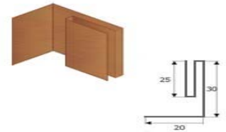
Планка завершающая для откоса
